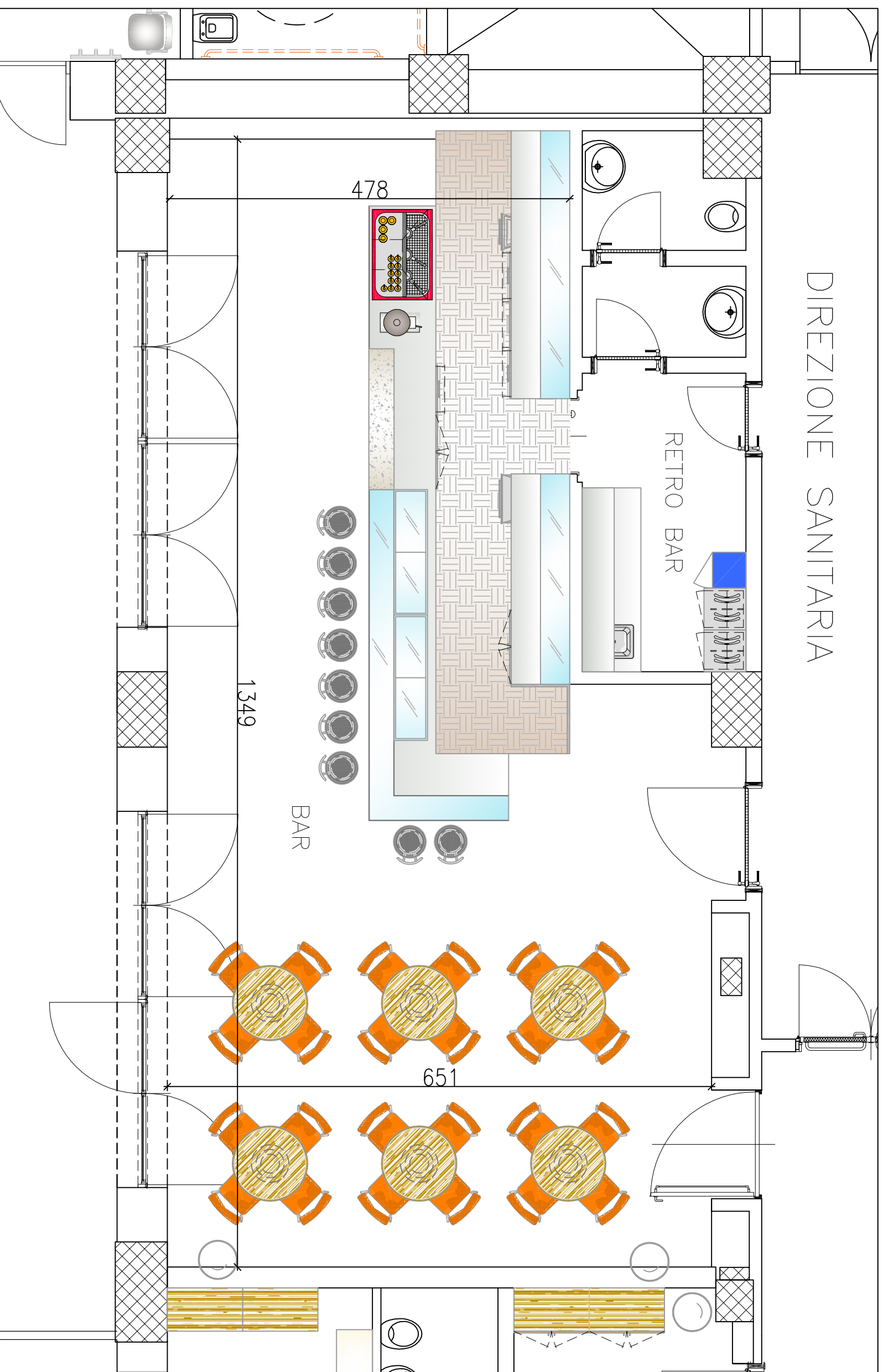
PLANIMETRIA AMBIENTE DENOMINATO "BAR" - PIANO RIALZATO - STRUTTURA OSPEDALIERA - SCALA 1:50
